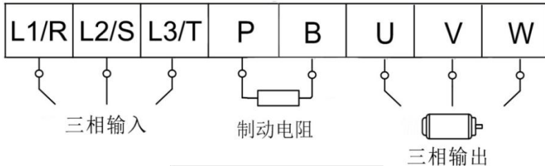
图 4-2 端子示意图
