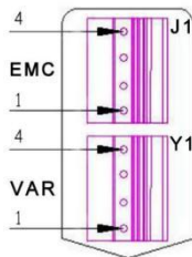
图 4-20 安规跳线接插件 J1、Y1 示意图
