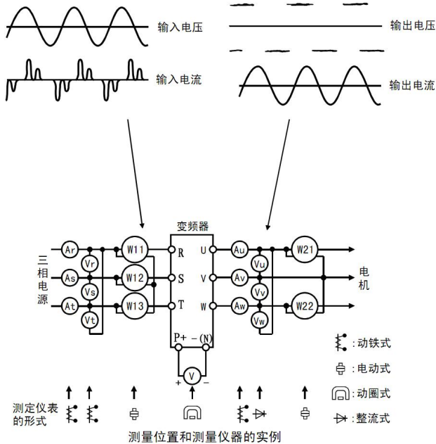
图 4-13 测量示意图
