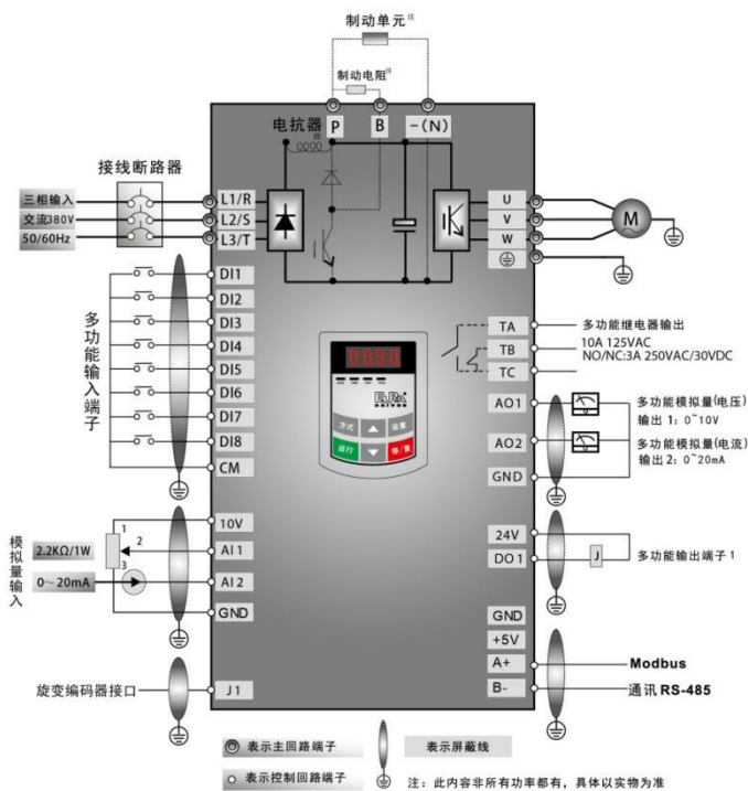
图 4-14 三相 T3 变频器标准配线图 (NPN 方式)
