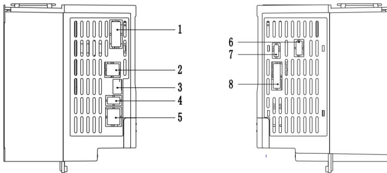
图 2-7 E2~E6 接口图
