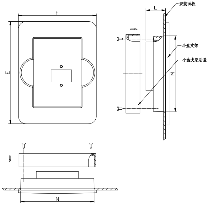
图 3-4 控制面板安装支架结构尺寸示意图
