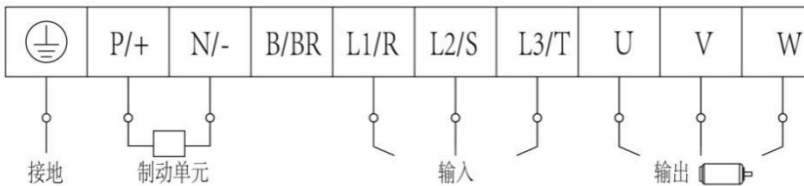
图 4-5 端子示意图
