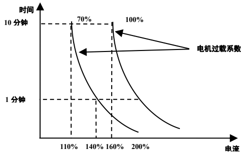
图 6-19 电机过载系数设定
