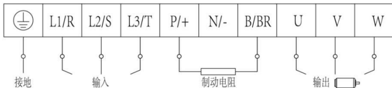
图 4-4 端子示意图
