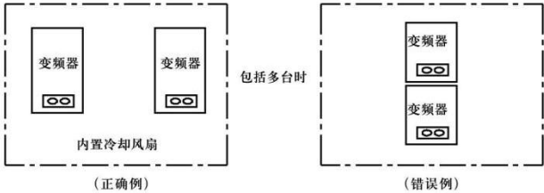
图 1-3 变频器安装在控制柜内示意图
