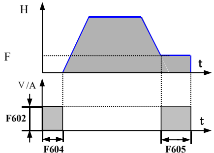
图 6-18 直流制动
