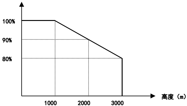
图 1-1 变频器额定电流与海拔高度降额曲线图
