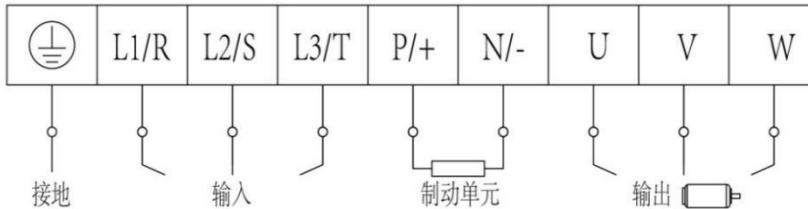
图 4-6 端子示意图
