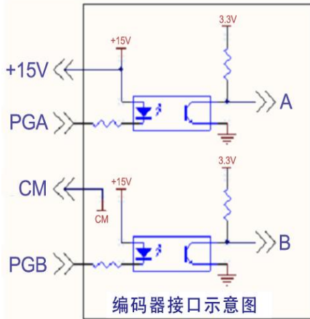
非差分输入编码器接口示意图
