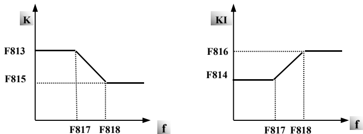
图 6-22 PI 参数示意图
