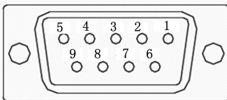
图 4-7 旋转变压器编码器端子排列示意图
