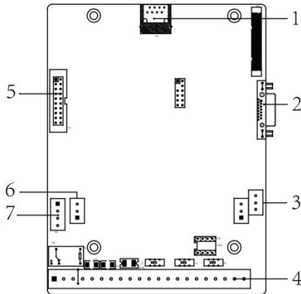
图 2-8 E7 及铁壳接口图
