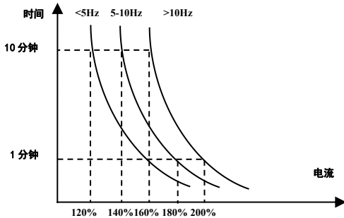
图 6-20 不同频率下的电机过载保护值
