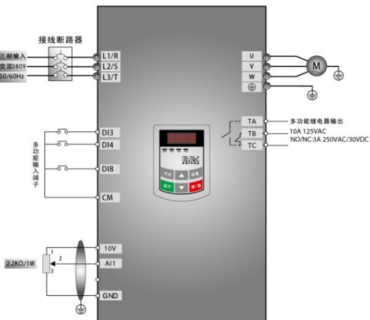
图 5-3 接线图 3
