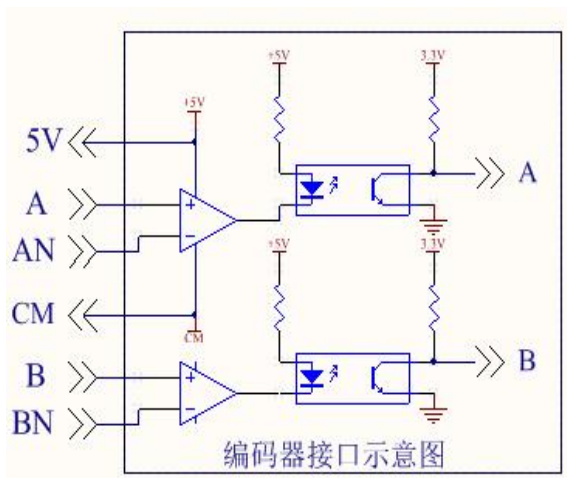
差分输入编码器接口示意图
