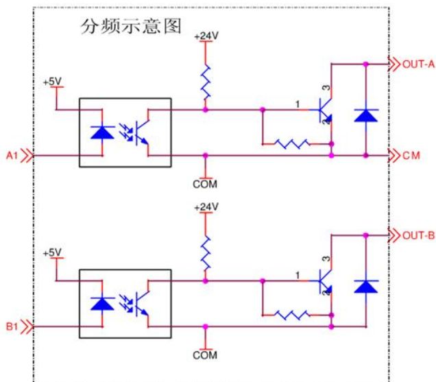
分频器接口示意图
